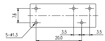
Schaltbild / Printbild
