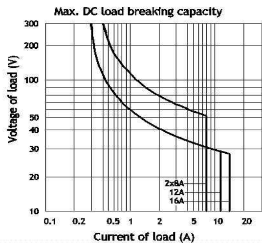
Gleichstrom - Lastgrenzkurve
