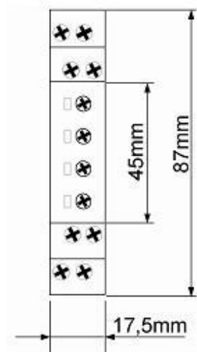
Ansicht auf Anschlüsse.
